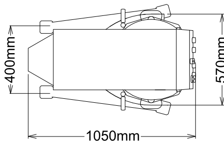
Felülnézet
